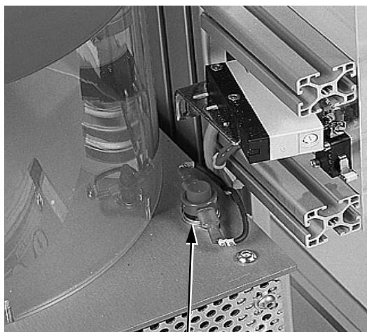
Thermorupteur de sécurité
