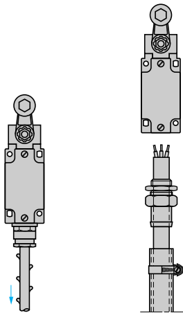
Position du presse étoupe
