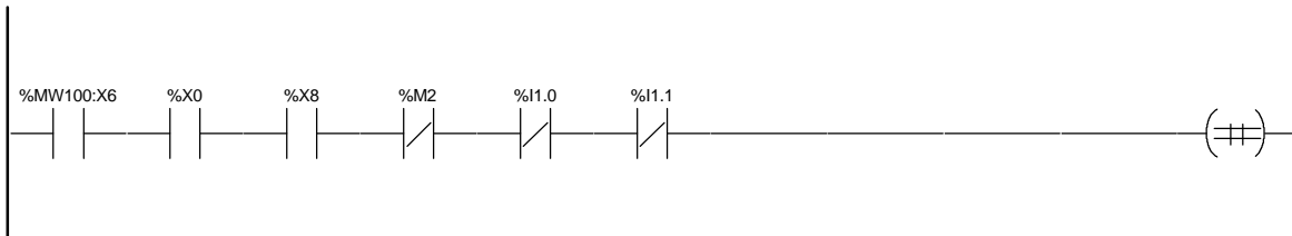
CHART - PAGE2 %X(16)->%X(17)
