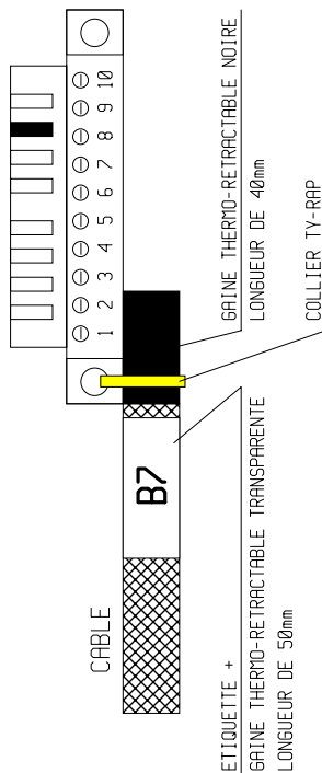
B7: CABLE 12xØ,6mm 2 DE LONGUEUR 5m SORTIE DE BOITE
