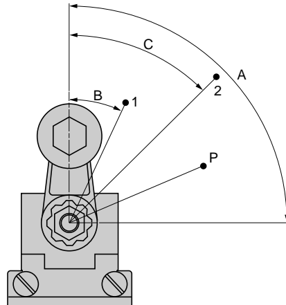
Mouvement angulaire
