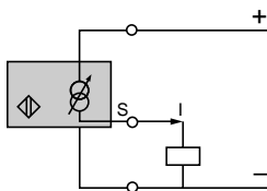
Branchement "3 fils"
